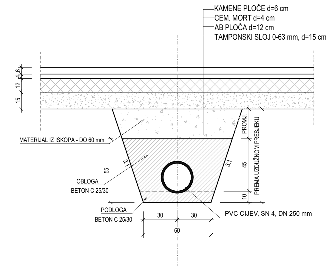
POPREČNI PRESJEK 1-1 OBORINSKE KANALIZACIJE PRIMORSKE ULICE KROZ OBALNI ZID MJ. 1:20
