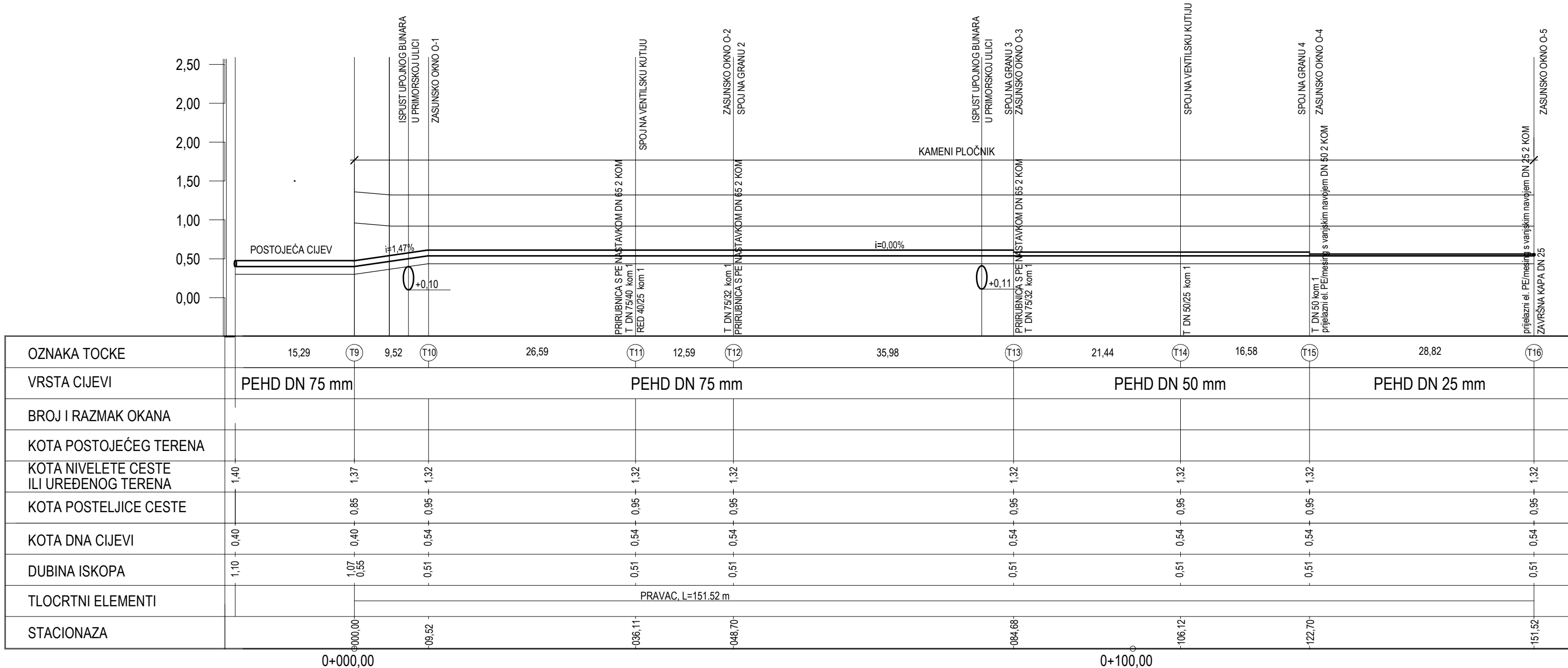
UZDUŽNI PROFIL GLAVNOG OPSKRBNOG CJEVOVODA-GRANA 1:
