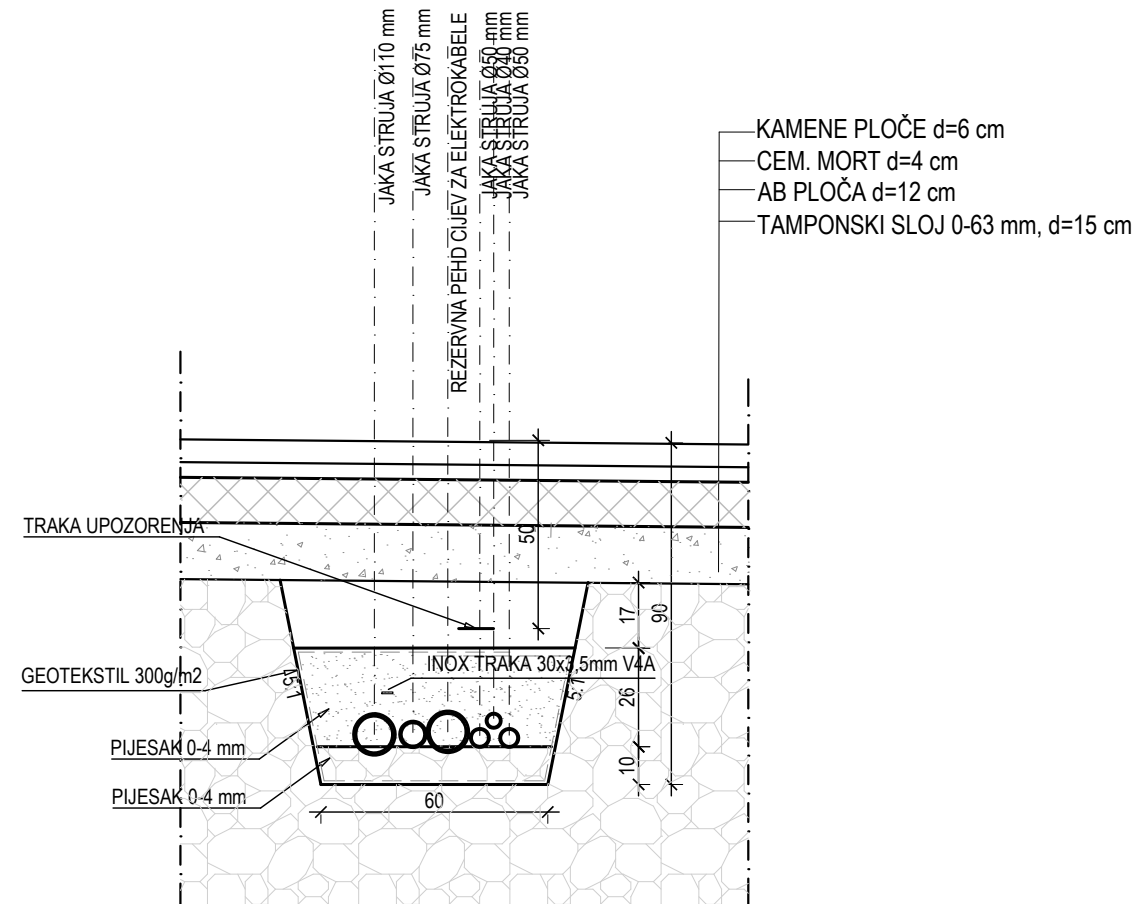
DETALJ ROVA ELEKTROINSTALACIJA I EKI INSTALACIJA
