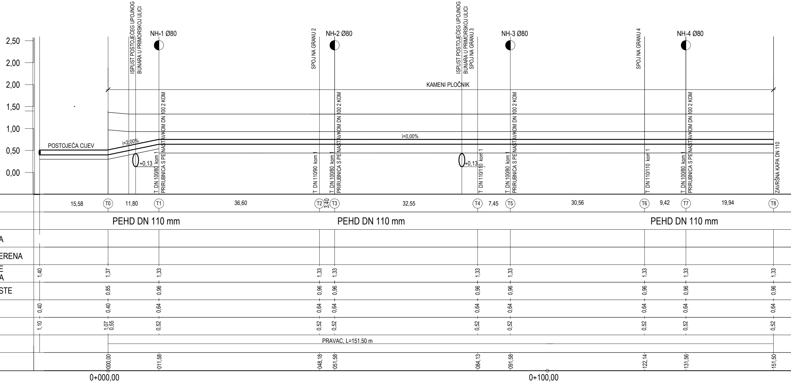
UZDUŽNI PROFIL HIDRANTSKOG CJEVOVODA- GRANA 1:
