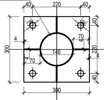
PRESJEK 1-1 MJ. 1:10
