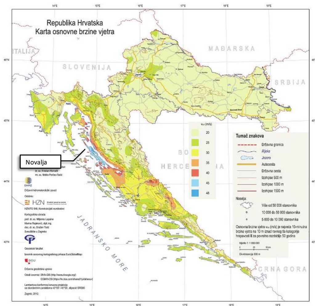
Slika 1(HR) – Osnovna brzina vjetra v_{b,0}
