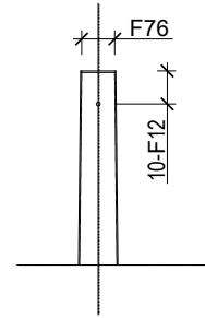
DETALJ A MJ. 1:10
